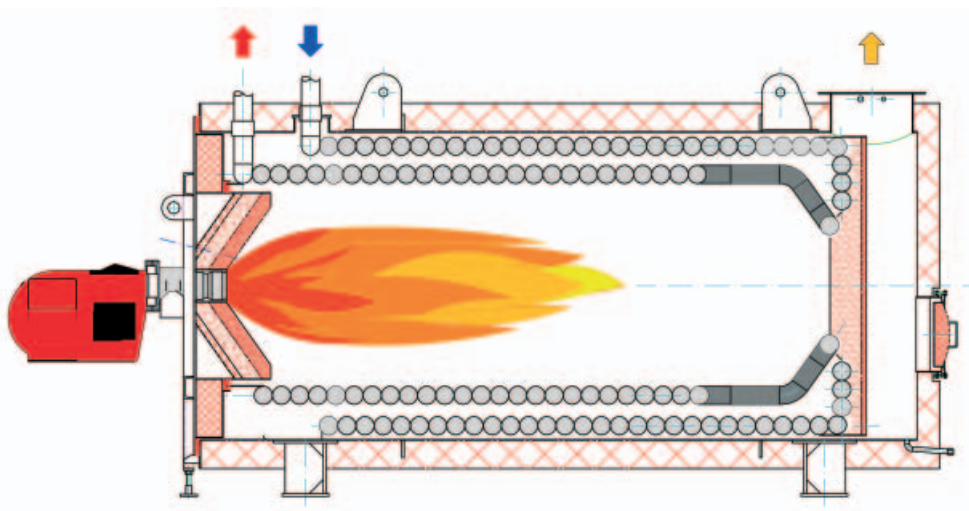
INTEC®-Thermalölerhitzer im Querschnitt
